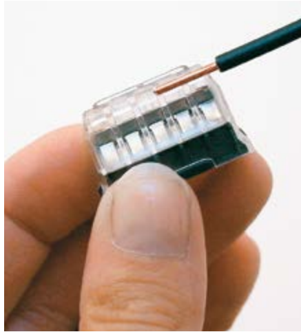
Leiter 8 – 9 mm abisolieren Strip wire 8 – 9 mm
