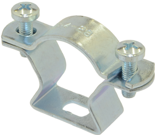
230.13.03Klem voor buis en kabelM25
