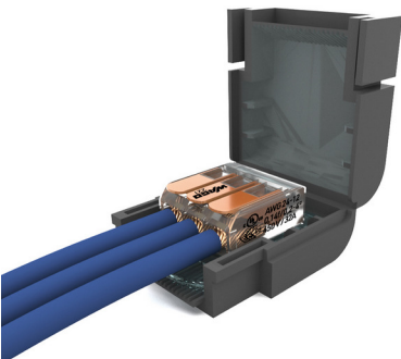
ShellBox 113 FLAT - WAGO 3 x 0,2-4mm² - 1pc per blister
