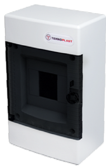
Verdeelkast opbouw - IP40 - 4 Modules235 x 139 x 98
