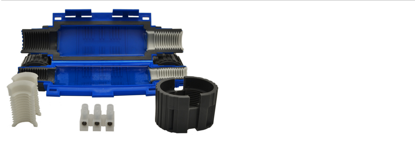
Rechte Koppeling gevuld met Gel - IP68 - 0.6/1 KVMet Connector - 3 polig, 3 x 6 mm²
