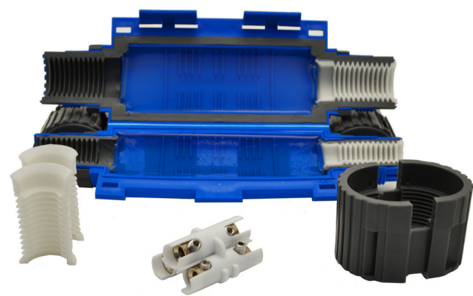
Rechte Koppeling gevuld met Gel - IP68 - 0.6/1 KVMet Connector - 5 polig, 2.5- 6 mm²
