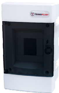
Verdeelkast Inbouw - IP40 - 4 Modules235 x 139 x 98
