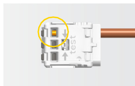
Controle opening voor inspectie van de gestripte en ingestoken geleider/fenêtre d'inspection pour vérification du dénudage et insertion.
