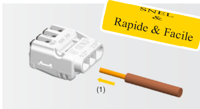
Voor éénaderige geleiders is het niet nodig de hendel te openen. Pour câbles rigides il n'est pas nécessaire d'ouvrir le levier.
