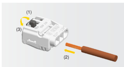
Voor flexibele geleiders hendel volledig openen/sluiten Pour câbles souples ouvrir/fermer levier entièrement.
